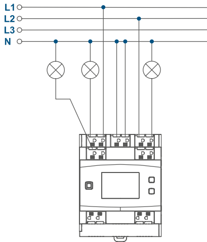
Zapojení stmívatelných světel (výstup):
