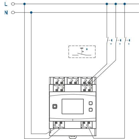
Zapojení tlačítek (vstup):
