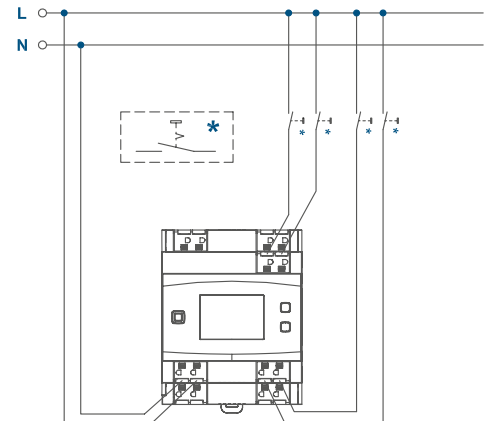
Připojení tlačítek/vypínačů (vstupů):
