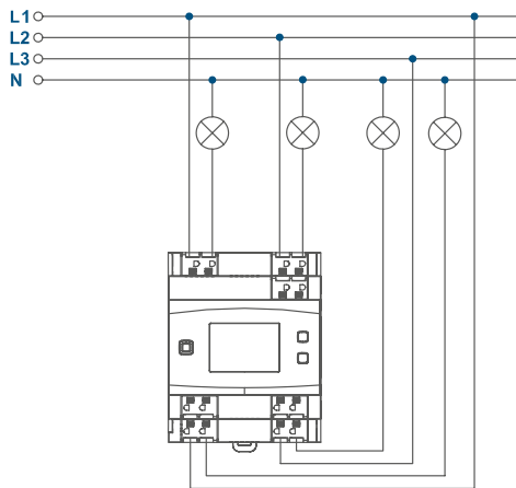
Připojení různých spotřebičů (výstupy):
